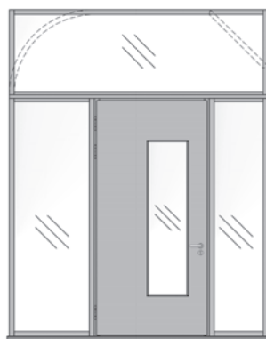
Sperrtürelement 1- flg. mit Seitenteilen, Oberlicht, Glasausschnitt
